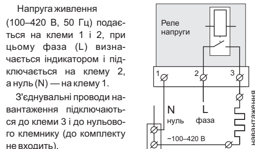
Схема 1. Спрощена внутрішня схема та схема підключення
