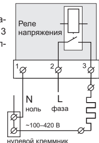
Упрощенная внутренняя схема и схема подключения
