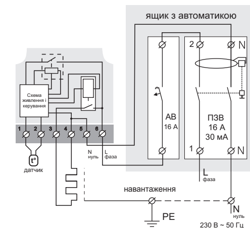
Схема 2. Підключення автоматичного вимикача і ПЗВ
