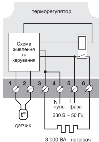
Схема 1. Схема підключення та спрощена внутрішня схема
