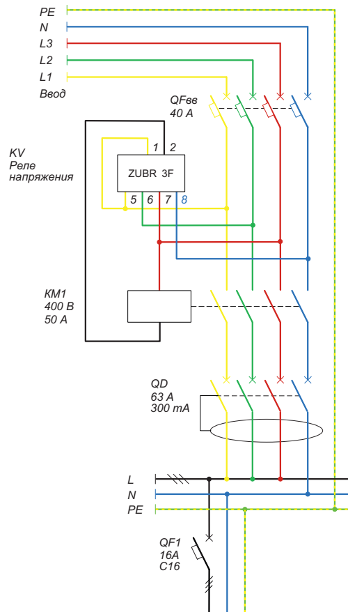
Схема 2. Вариант электрической схемы ZUBR 3F и контактора с обмоткой на 400 В
