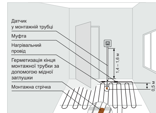
Рисунок 1. Монтаж терморегулятора та теплої підлоги
