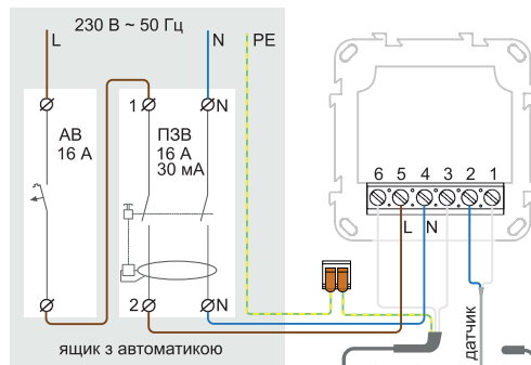
Схема 1. Підключення термостата для обігріву двожильним кабелем
