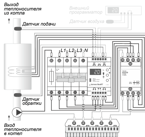
Схема 2. Подключение автоматики 3-х фазного котла
