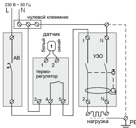
Схема 2. Подключение АВ и УЗО
