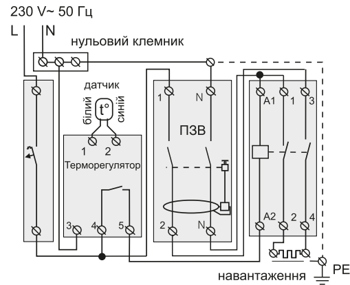
Схема 2. Підключення через контактор (магнітний пускач)
