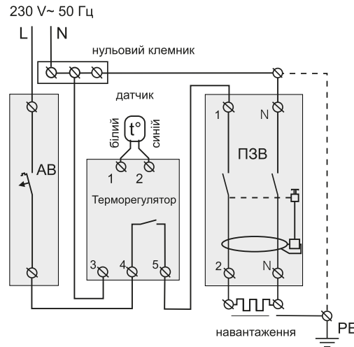
Схема 1. Схема підключення терморегулятора, автоматичного вимикача і ПЗВ
