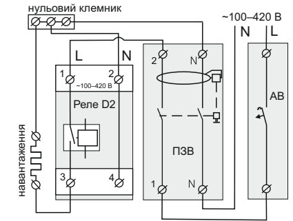
Схема 2. Підключення автоматичного вимикача та ПЗВ без транзита нуля через реле
