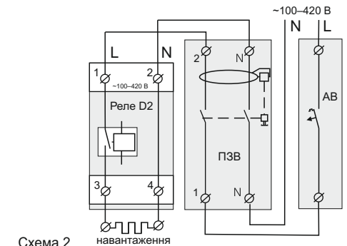
Схема 2. Підключення автоматичного вимикача та ПЗВ
