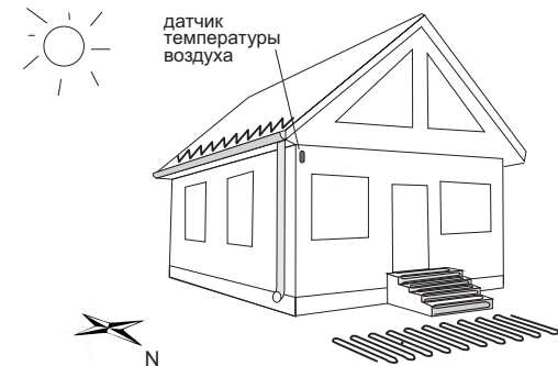
Рисунок 1. Монтаж датчика температуры воздуха
