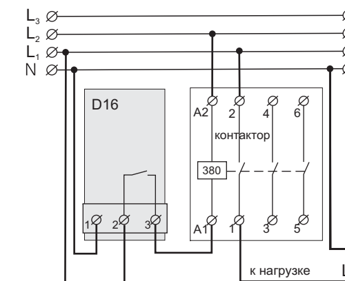
Схема 4. Подключение реле напряжения и контактора с обмоткой 380 VAC
