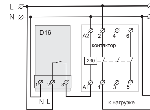
Схема 3. Подключение реле напряжения и контактора с обмоткой 230 VAC
